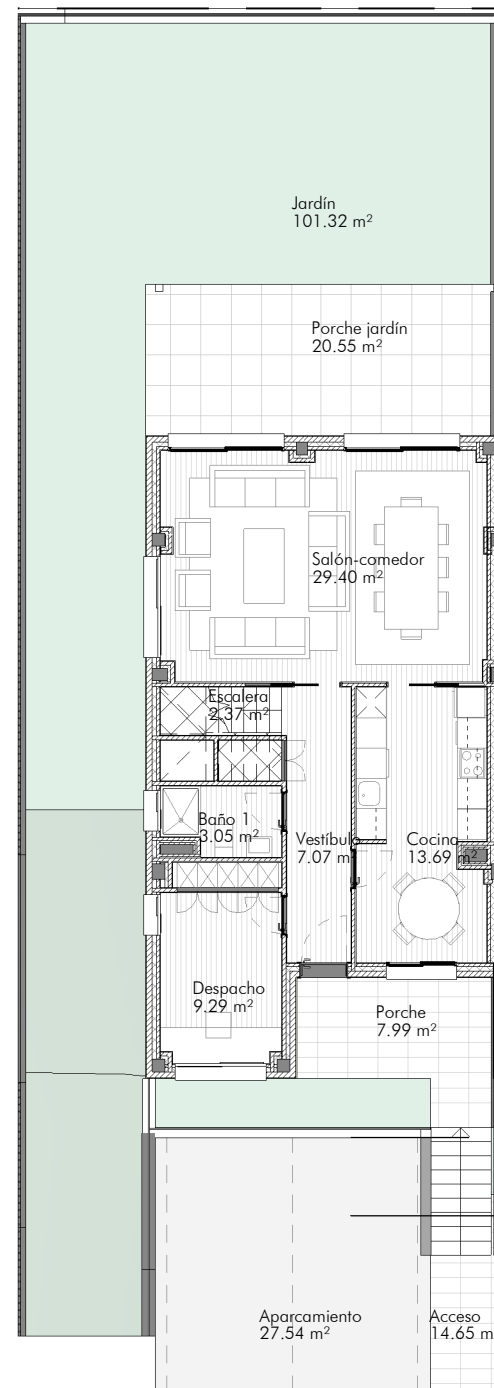
PLANTA BAJA 1 : 150
