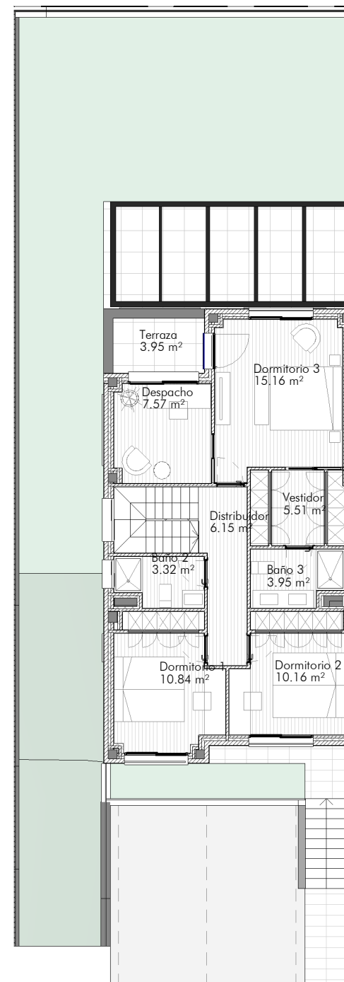
PLANTA PRIMERA 1 : 150
