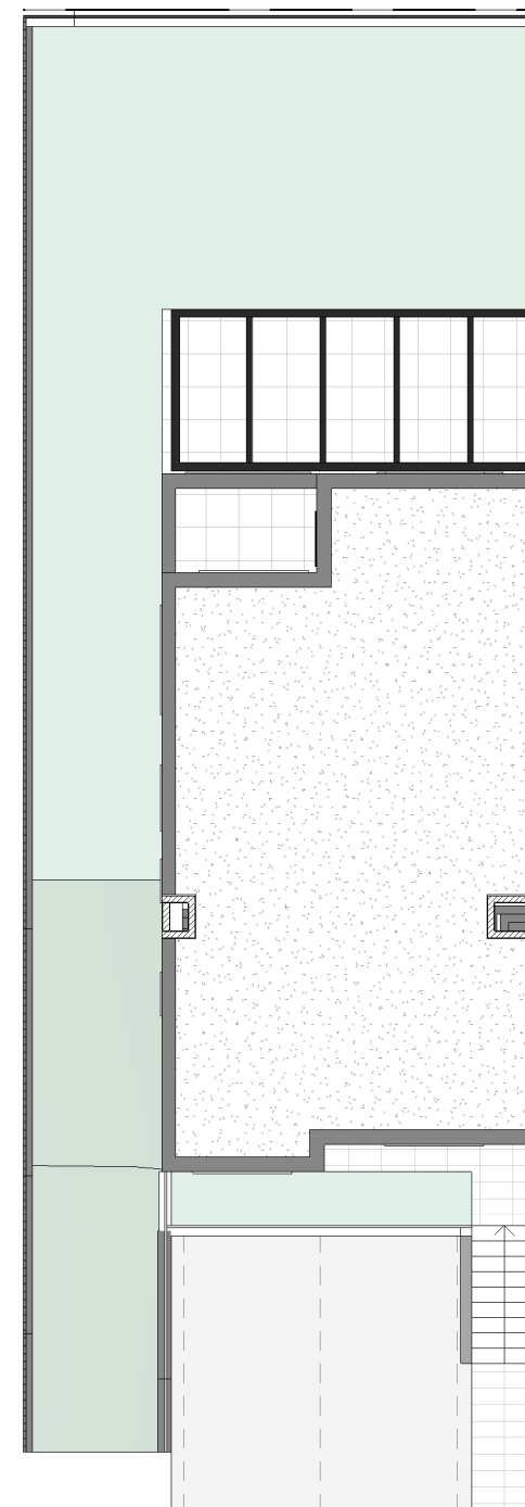
PLANTA CUBIERTA 1 : 150
